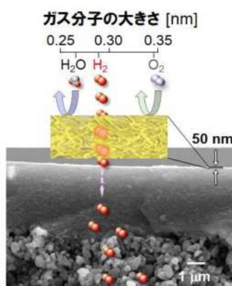
開発中の水素分離膜
